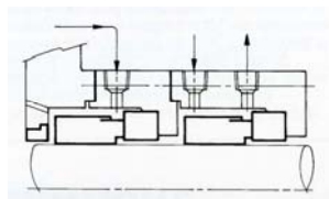
Двойное уплотнение тандем
