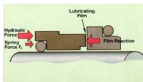
Силы, действующие на уплотнение
